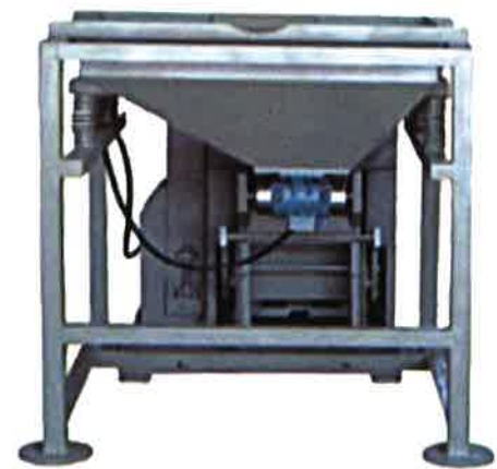
Eccentric Motor Type 此款儲料桶採用偏心馬達裝置
