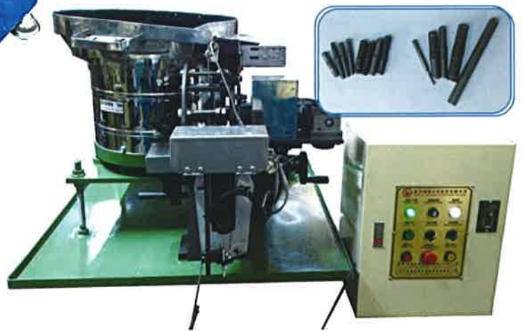
款式二 Vertical Type 立式
