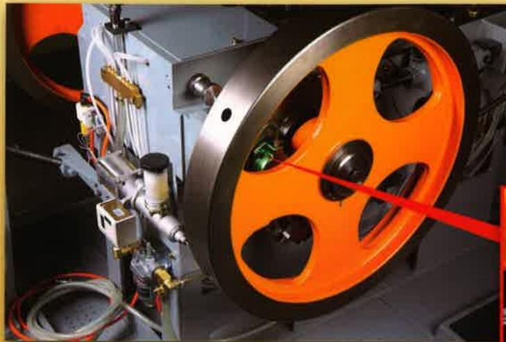
煞車系統 AIR BRAKE SYSTEM
